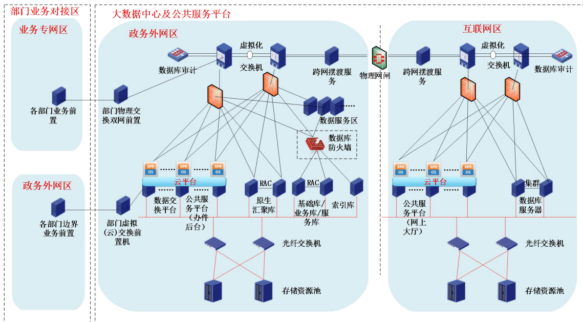
图 1 平台网络总体拓扑图
