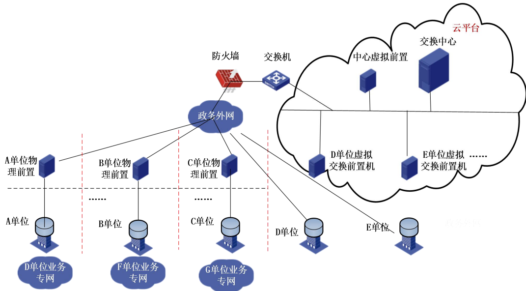
图 2 各单位对接网络拓扑图
