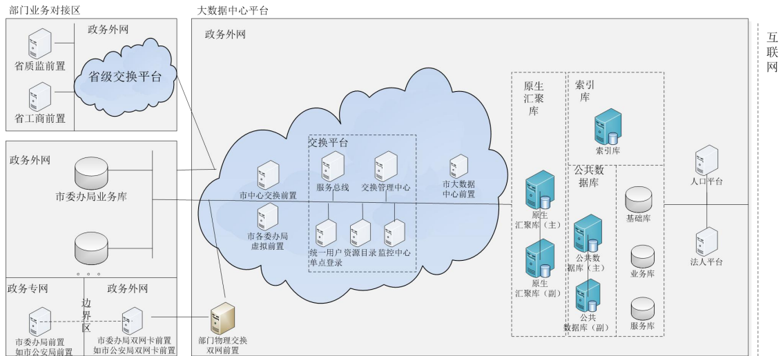
图 3 大数据中心平台部署图
